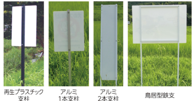
取付例 [背面より撮影]
